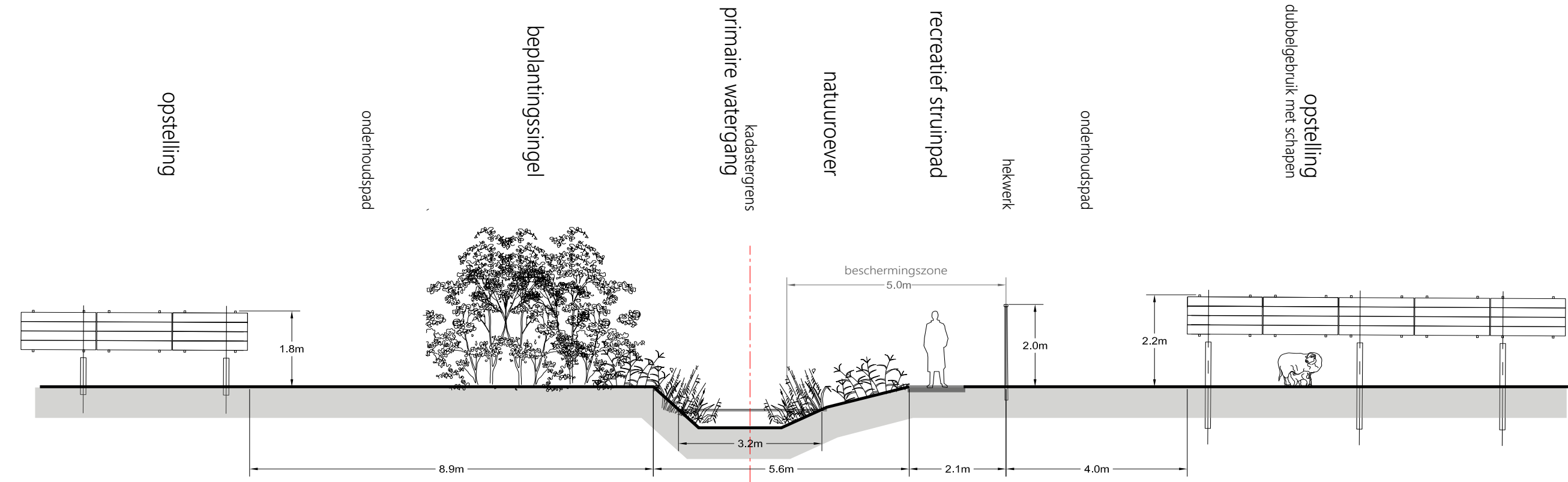
Profiel 3 schaal 1:100
