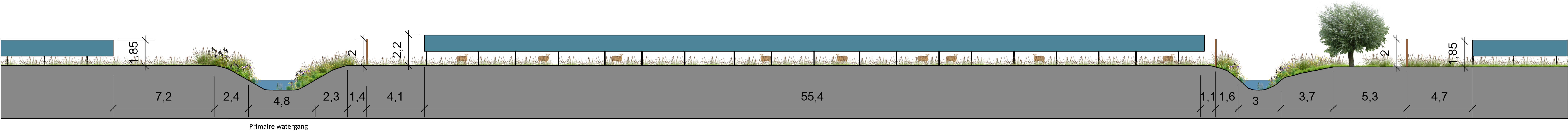
Profiel 1
